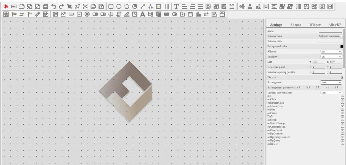
Рисунок 1 – Редактор виджетов
