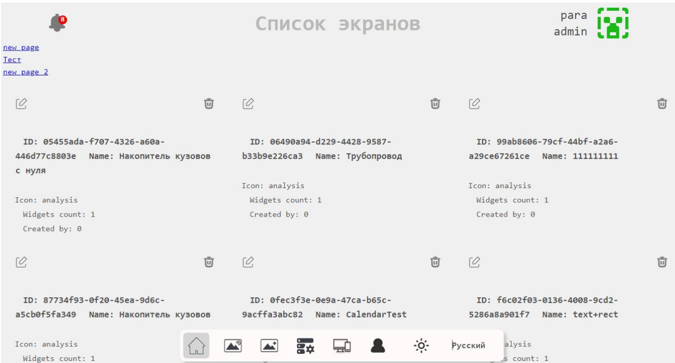
Рисунок 7 – Светлая тема
