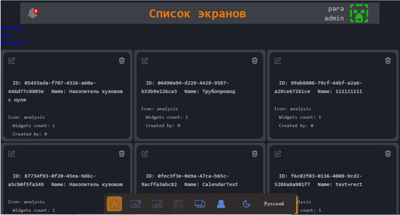
Рисунок 8 – Темная тема
