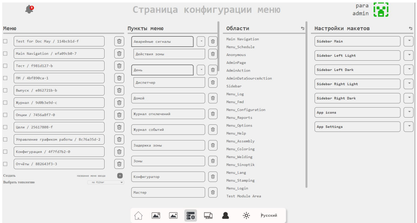
Рисунок 3 – Конфигуратор интерфейса
