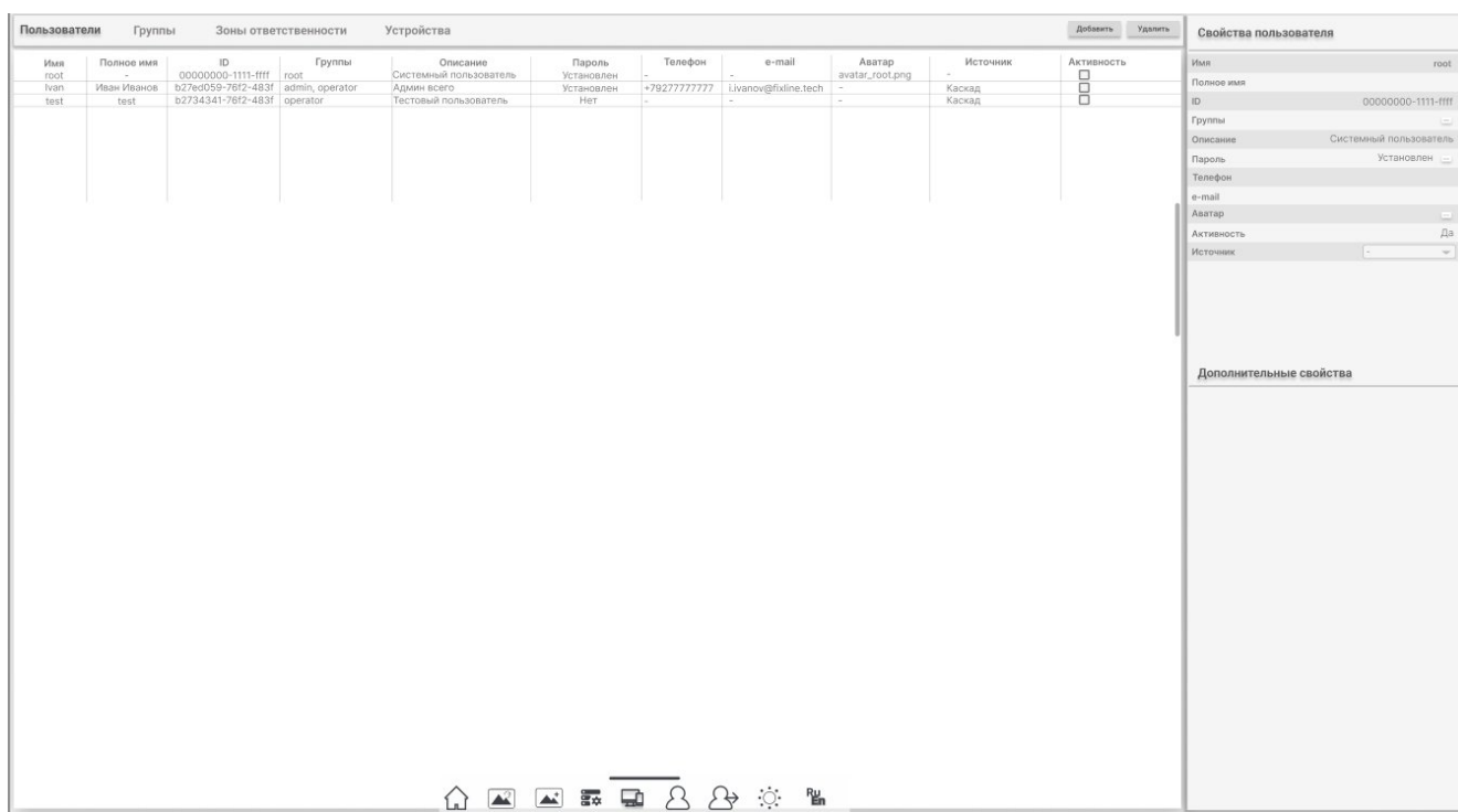
Рисунок 6 – Пользователи
